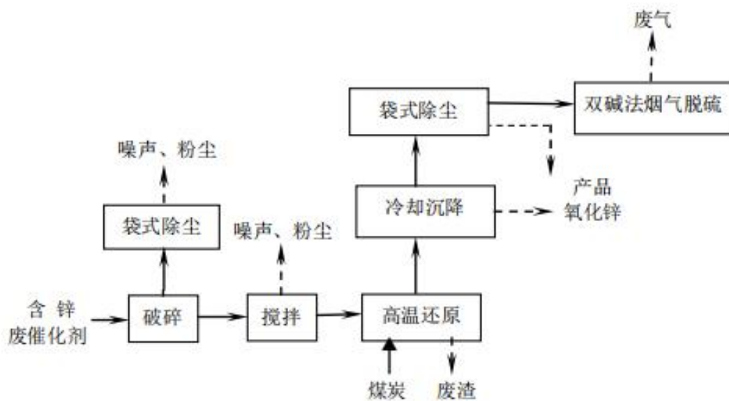
图 3.5-3 含锌废催化剂提取工艺流程及产污环节
