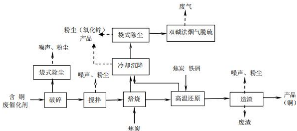
图 3.5-2 含铜锌废催化剂提取工艺流程及产污环节
