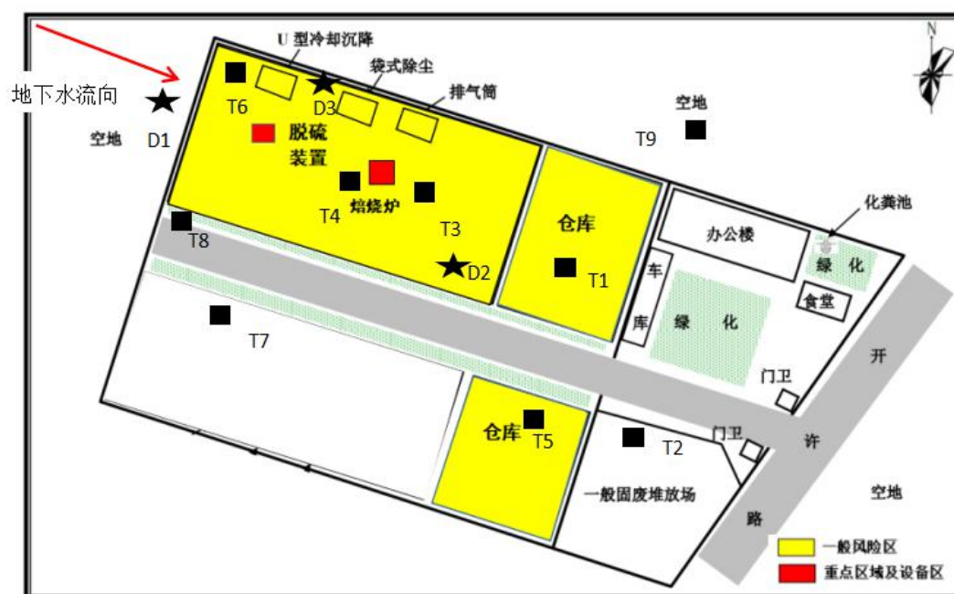
图 5-1 为土壤地下水采样点位布设示意图图
