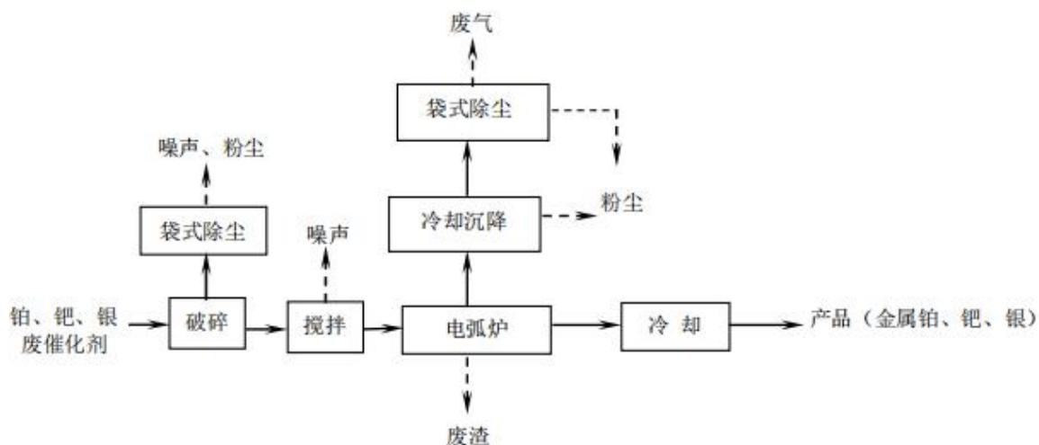
图 3.5-4 含铂、钯、银废催化剂提取工艺流程及产污环节
