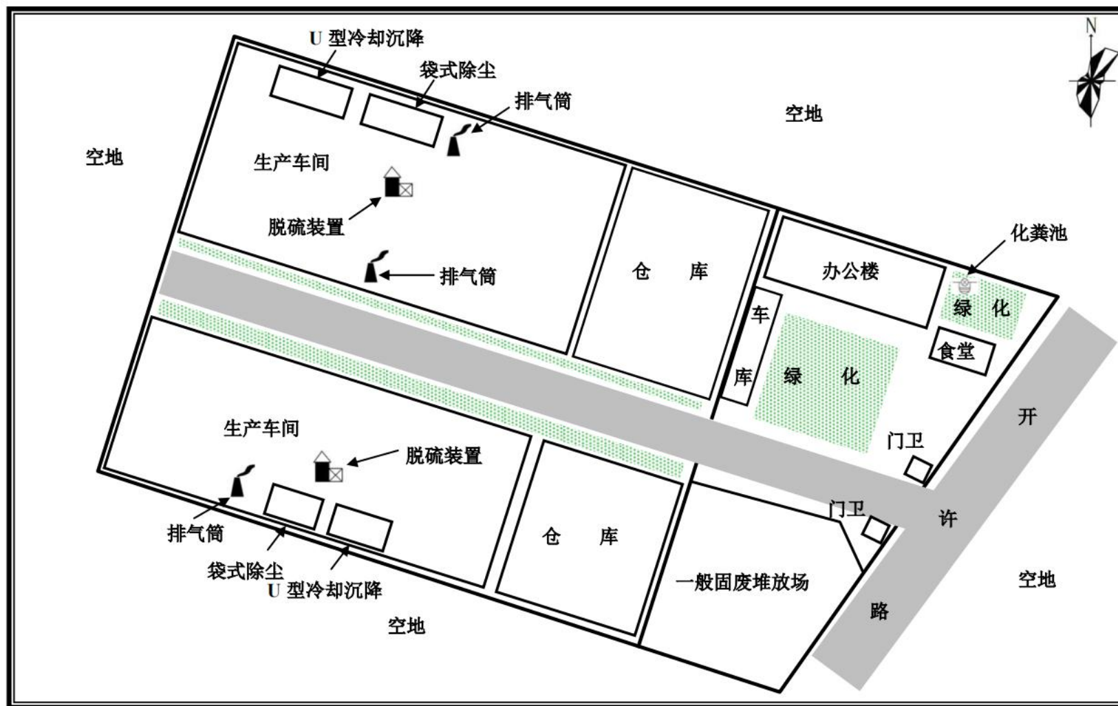
图 3-2 尉氏县豫达有色金属有限公司厂区平面布置图
